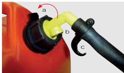
Kanister 25l mit Zapfpistolenpumpe
