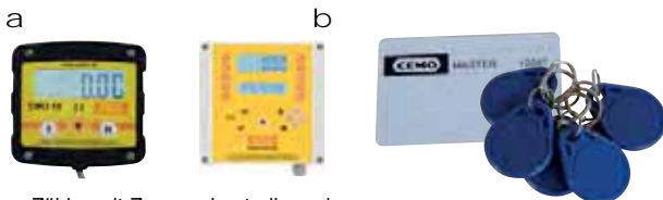
a Zähler mit Zugangskontrolle und Tankdaten-Verwaltungssystem „CMO 10“ für bis zu 250 Benutzer
