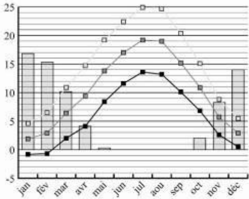
Courbe des températures et jours avec gelée sous abri période 1980 - 2009
