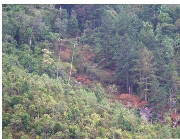
Foto 81 e 82- Processo de escorregamentos planar, erosão laminar e em sulcos, freqüentes e de média a alta intensidade e soterramento no fundo do vale que caracterizam os Terrenos Montanhosos e Escarpados.
