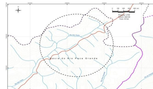
FIGURA C – Trecho amostral de padrão treliça nas cabeceiras do rio Paca Grande
