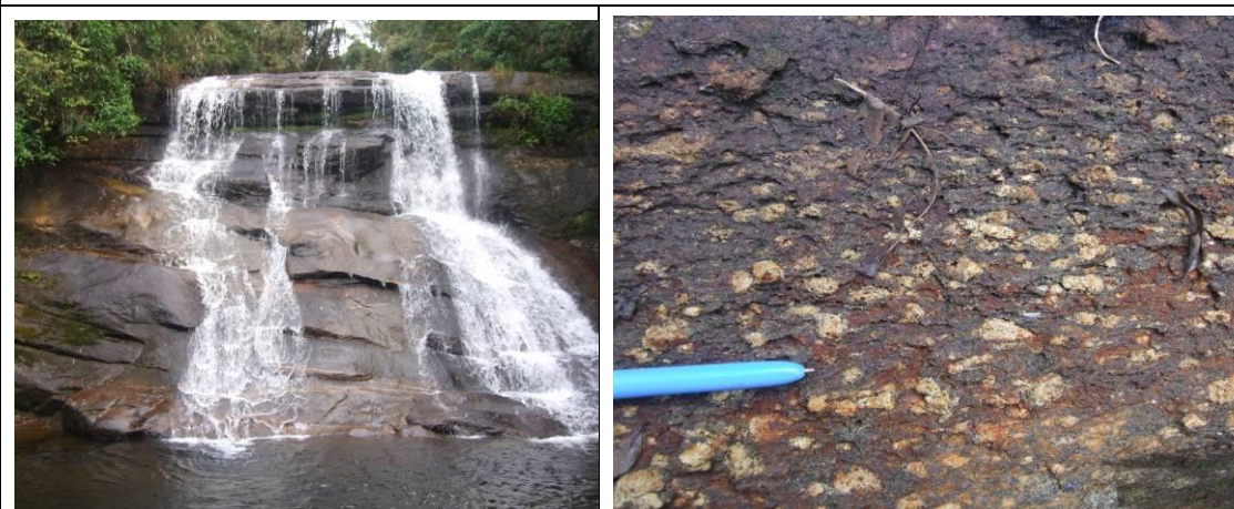
Fotos 73 e 74 – Queda 6 da Cachoeira Sete Quedas no Rio do Braço, sustentada por Hornblenda-biotita gnaíse migmatítico com porfiroblastos de plagioclásio do Complexo Quirino, nos Terrenos Montanhosos e Escarpados. 286 / 290 (23 K 564815 7478021)
