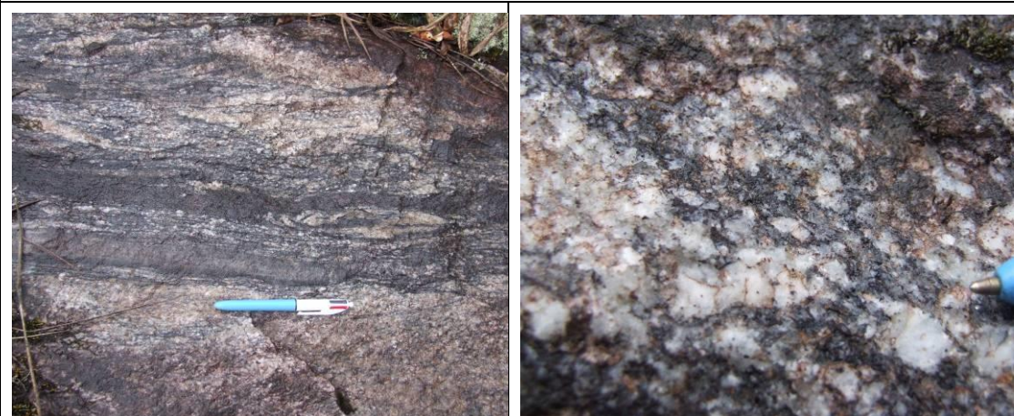
Foto 69 e 70 - Hornblenda-biotita gnaíse migmatítico, leuco a mesocráticos, de granulometria variando de média à grossa, com foliação descontínua marcada por aglomerados minerais de hornblenda e enclaves máficos alongados, do Complexo Quirino, que sustenta o relevo de Montanhas e Morros que caracteriza os Terrenos Montanhosos e Escarpados. 100 /102 (23 K 563864 7478648)
