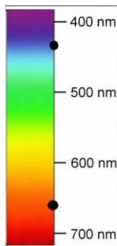
Abbildung 9: Lichtspektrum
