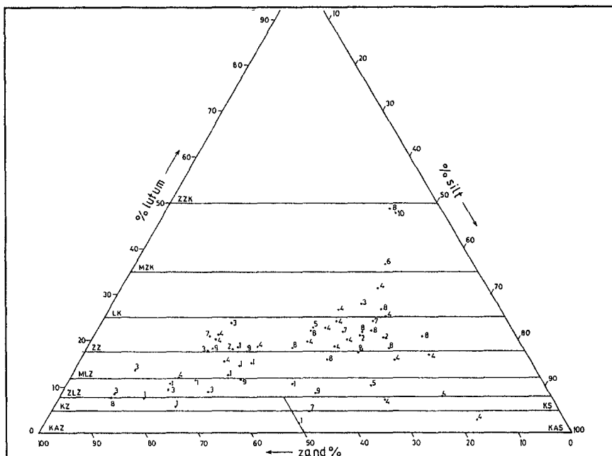
Figuur 3.4 Zand-silt-lutumdriehoek met opnamen en clusternummers.
