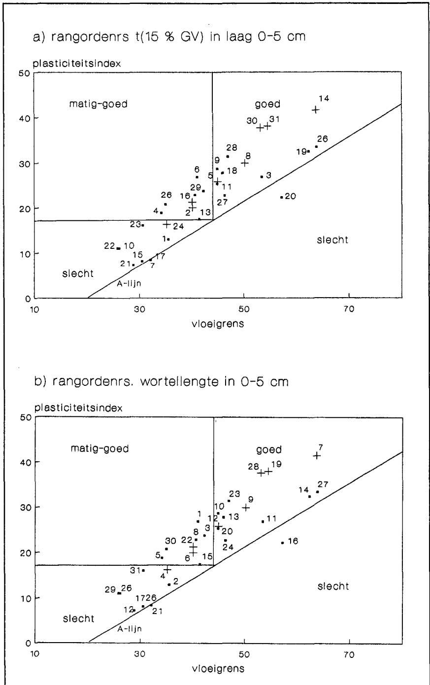
Figuur 6.12 Plasticiteitsdiagram met rangordennummers volgens oplopen- de erosiecentrifugetijd (a) en wortellengte (b).
