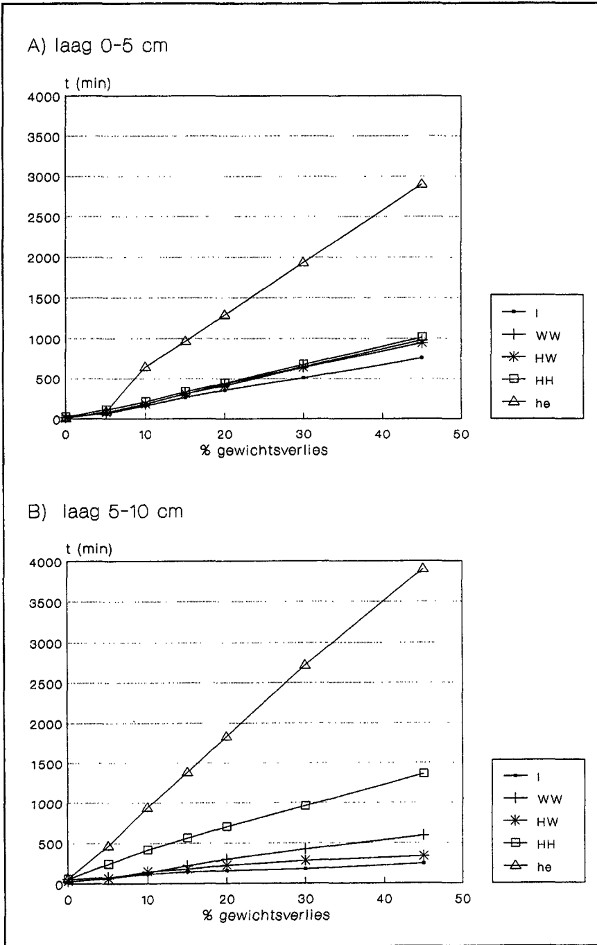
Figuur 6.9 Verband erosiecentrifugetijd - % gewichtsverlies in laag 0-5 cm (A) en 5-10 cm voor bemest weiden (l) en onbemest weiden (WW), hooien + weiden (HW), hooien (HH) en langdurig onbemest hooien (he)
