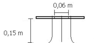
Detail invliegopening met anti-uitvlieg stangetjes (zijaanzicht)
