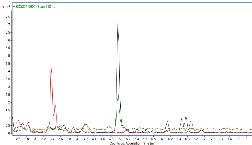
Sorbus paxiana
